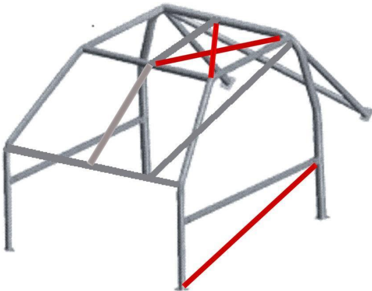
Voorbeeld kooiconstructie:
